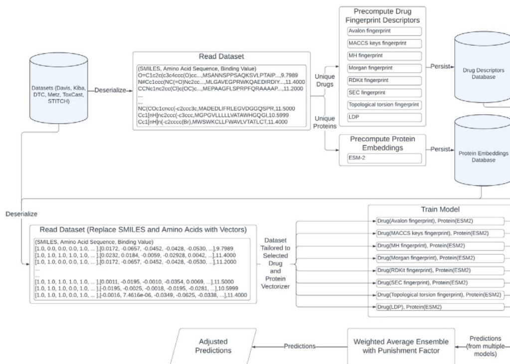
图 4.WAE-DTI 架构。首先，我们遍历每个数据集并提取独特的药物和蛋白质。对于每种药物，我们使用多种描述符计算其特征表示，包括原子对指纹、Avalon 指纹、MACCS 密钥指纹、MH 指纹、Morgan 指纹、RDKit 指纹、SEC 指纹、拓扑扭曲指纹和 LDP。对于每种蛋白质，我们使用 ESM-2 计算其嵌入。所有特征都通过存储在磁盘上来持久化。在训练过程中，我们使用计算出的特征来替换原始的 SMILES 表示和氨基酸序列。然后，我们对每个描述符进行排列，并训练其独立模型。根据模型在验证集上的表现，我们采用带有惩罚因子的加权平均集成，表现良好的模型会得到奖励；相反，表现不佳的模型会受到惩罚。集成模型的输出被视为最终预测结果。
